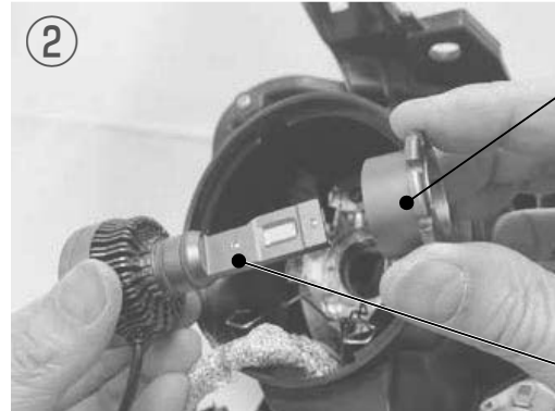
② LEDバルブのフランジ部をバルブから取外してください。
