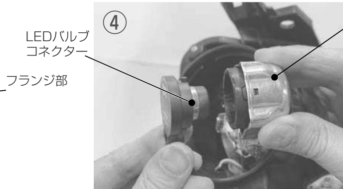
④ 純正HIDバラストコネクタとLEDバルブコネクタを接続し、ロック方向に回転させヘッドライトユニット可動域の邪魔にならない位置に付属の両面テープなどでコネクタを固定してください。
