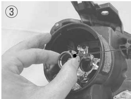
③ 取外したバルブフランジ部を、ヘッドライトユニットのバルブ取り付け部に固定してください。
