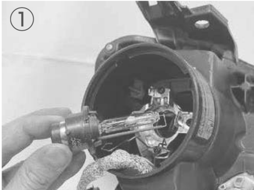
① 純正HIDバルブから純正HIDバラストコネクタを取外し、純正HIDバルブを取外してください。
