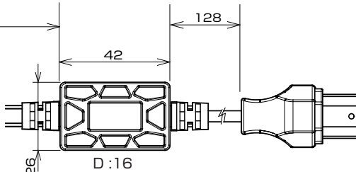
○ドライバー寸法
