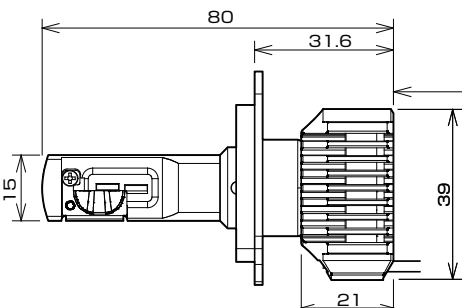
○LEDバルブ寸法
